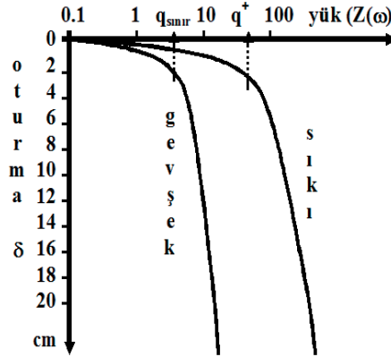
Şekil-7. Zeminlerin yük - oturma veya sismik empedans - deformasyon ilişkisi grafiği .
