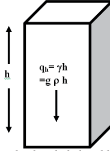
Şeki- 3. Birim alan kesitli, h derinlikli zemin sütunu
